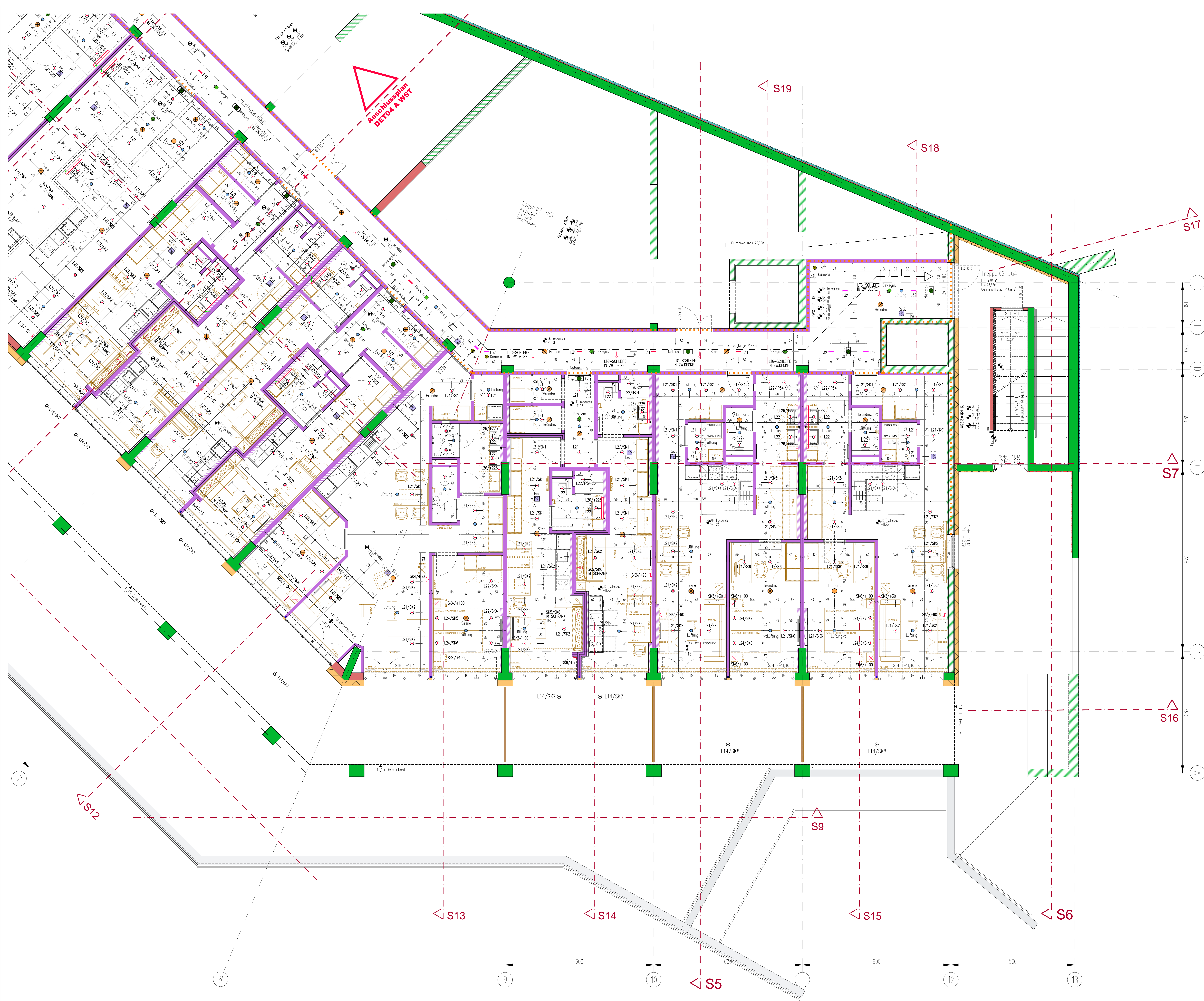
DECKENSPIEGEL UG4 OST - 1:50
